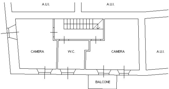
PIANO PRIMO H = 2.70 m
